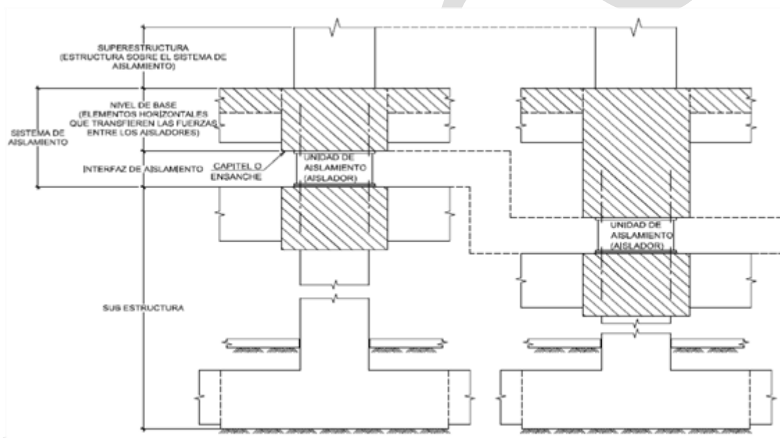
Figura N°1: Sistema de aislamiento sísmico
